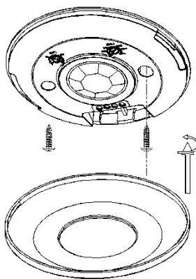
Рис. 2 Схема монтажа
