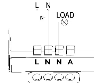
Рис. 3 Схема электропитания
