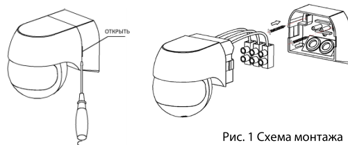
Рис. 1 Схема монтажа
